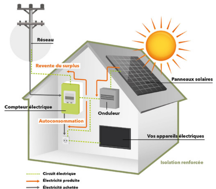
Schéma du fonctionnement d'une maison à énergie positive
